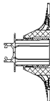
COUPE A-A
