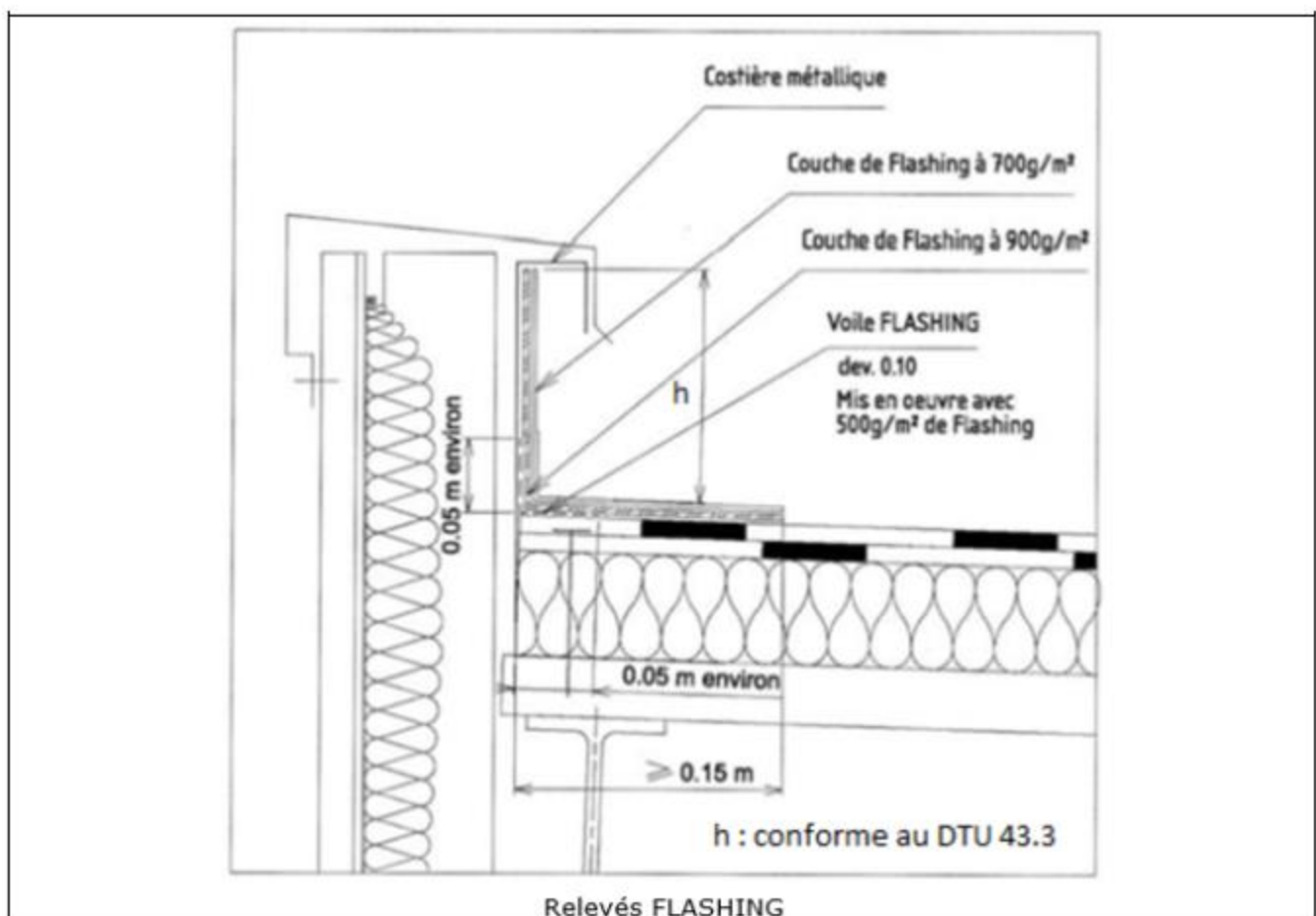
Figure 29 : Relevés en feuilles bitumineuses ou Flashing
