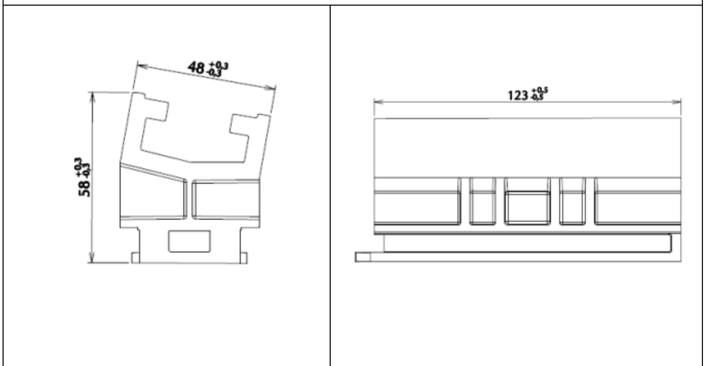
Figure 19 : Plan Réhausse 45 polymère
