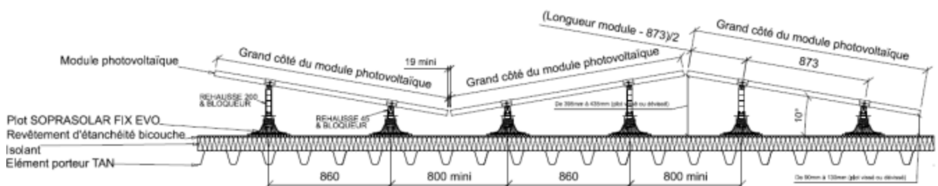
Figure 6 : Vue en coupe (dans le sens de la longueur des modules) du procédé avec modules photovoltaïques de longueur 1 755 mm en inclinaison double shed – rehausses aluminium
