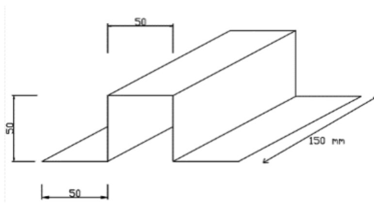
Figure 20 : Plots FIX EVO supports de chemin de câble
