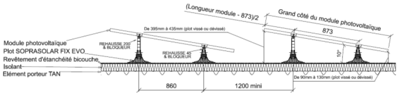
Figure 7 : Vue en coupe (dans le sens de la longueur des modules) du procédé avec modules photovoltaïques de longueur 1 755 mm en inclinaison simple shed – rehausses aluminium
