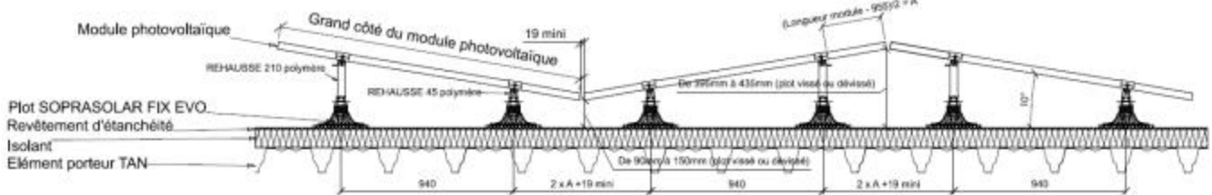
Figure 8 : Vue en coupe (dans le sens de la longueur des modules) du procédé avec modules photovoltaïques de longueur 1755mm en inclinaison double shed – rehausses polymère
