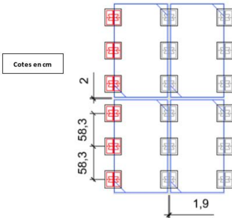
Figure 35 : Implantation des plots SOPRASOLAR FIX EVO en calepinage densifié
