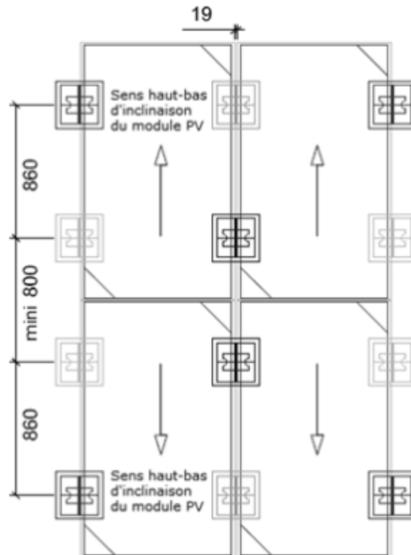
Figure 31 : Implantation des plots SOPRASOLAR FIX EVO avec modules photovoltaïques en inclinaison double shed
