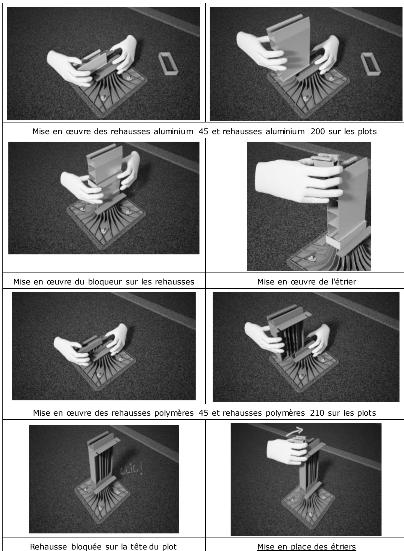
Figure 38 : Mise en œuvre des rehausse et bloqueurs et des étriers
