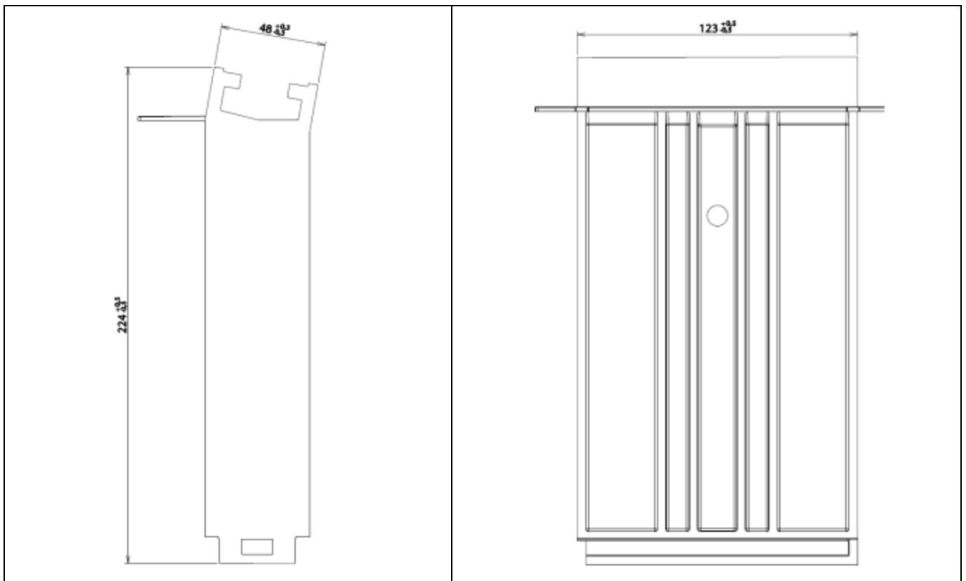
Figure 18 : Plan Réhausse 210 polymère – diamètre du perçage 9mm
