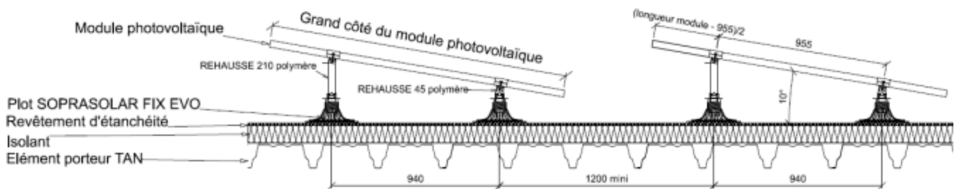
Figure 9 : Vue en coupe (dans le sens de la longueur des modules) du procédé avec modules photovoltaïques de longueur 1755mm en inclinaison simple shed – rehausses polymère
