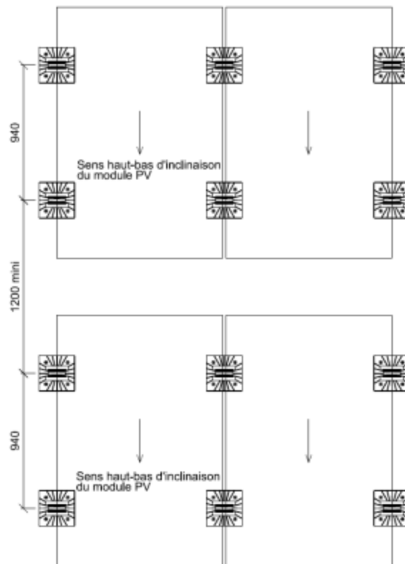
Figure 32 : Implantation des plots SOPRASOLAR FIX EVO avec modules photovoltaïques en inclinaison simple shed – rehausse polymère
