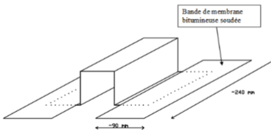
Figure 21 : Supports de chemin de câble par oméga
