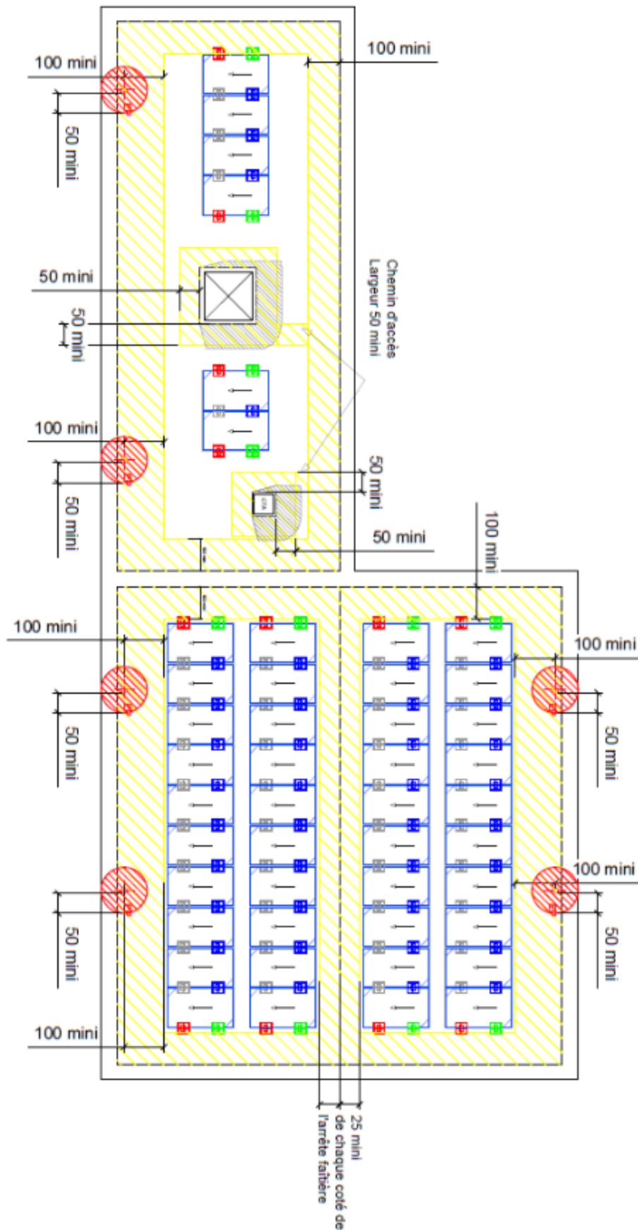
Figure 44 : Exemple calepinage et préparation de la toiture avec modules photovoltaïques inclinés en orientation simple shed
