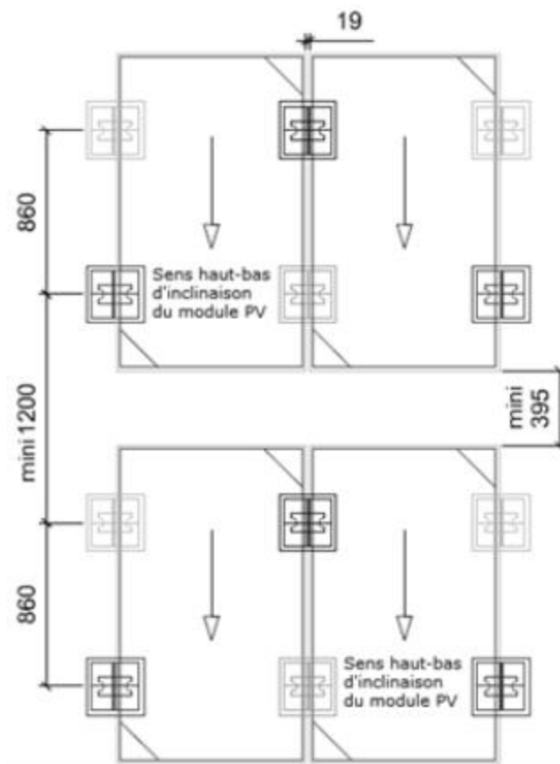
Figure 30 : Implantation des plots SOPRASOLAR FIX EVO avec modules photovoltaïques en inclinaison simple shed
