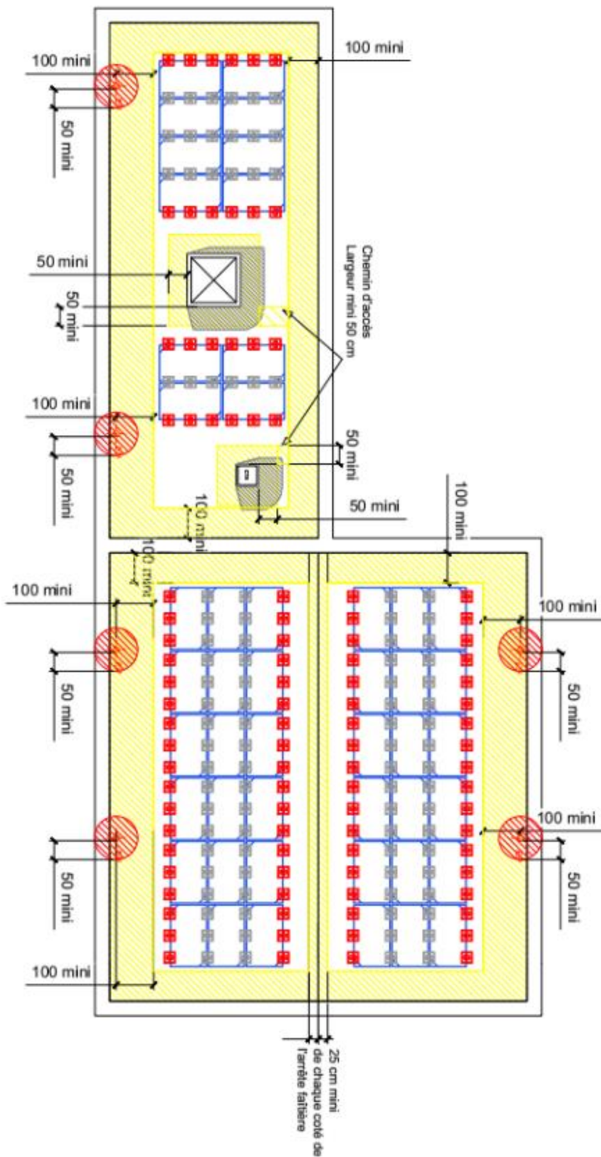
Figure 42 : Exemple calepinage standard (3 plots/grand côté du module) et préparation de la toiture en pose à plat
