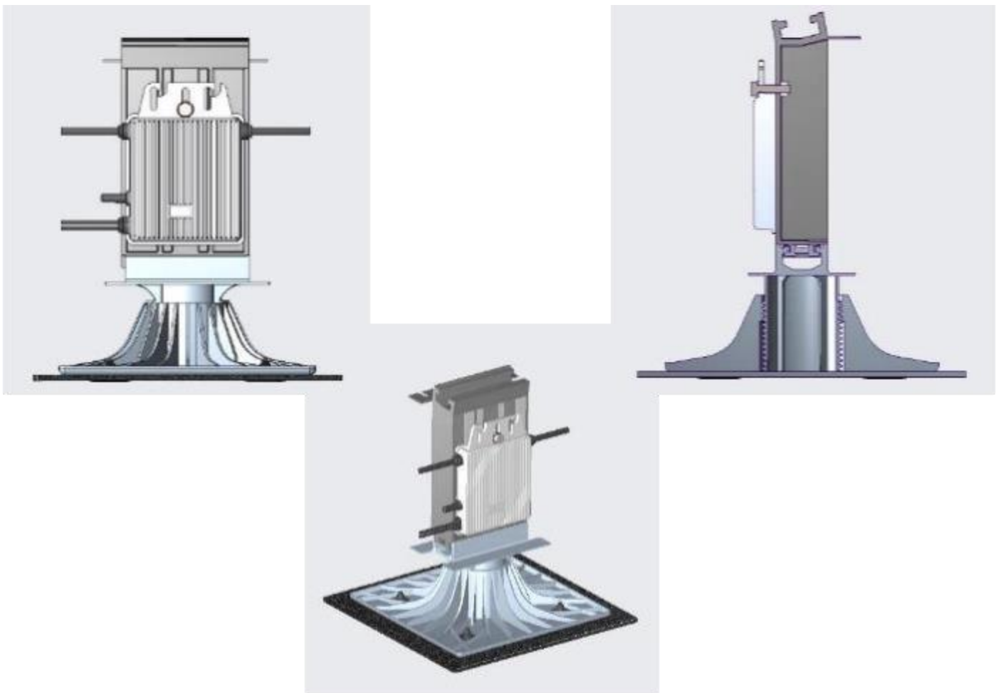
Figure 27 : Mise en place micro onduleur sur réhausse polymère – diamètre du perçage 9mm
