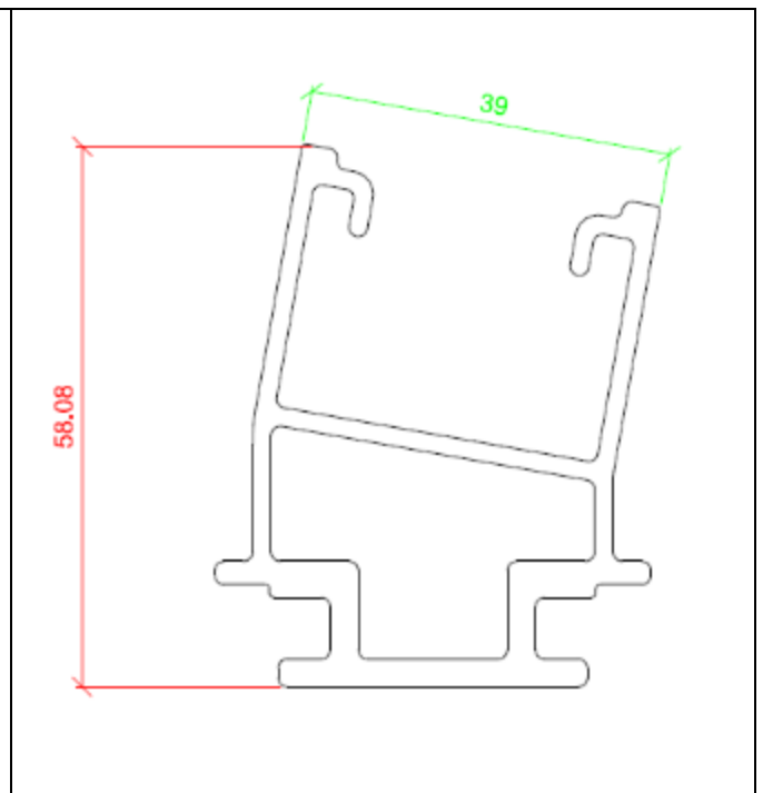
Figure 15 : Plan Réhausse 45 aluminium
