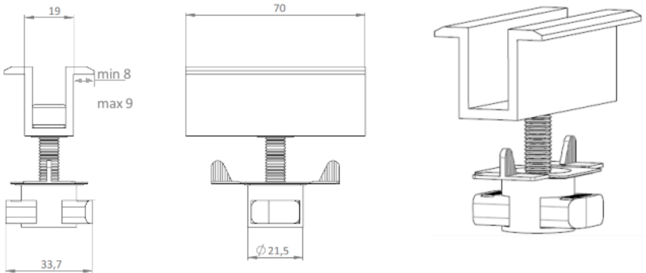
Figure 11 : Étrier intermédiaire
