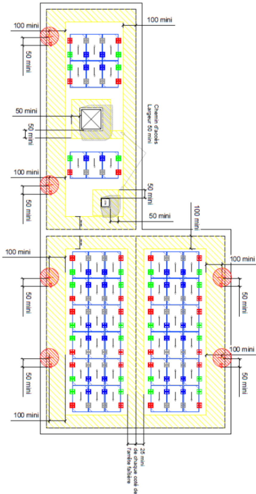
Figure 43 : Exemple calepinage et préparation de la toiture avec modules photovoltaïques inclinés en orientation double shed
