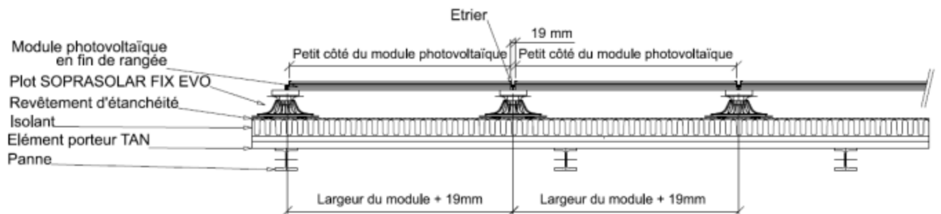
Figure 5 : Vue en coupe (dans le sens de la largeur des modules) du procédé avec modules photovoltaïques parallèles au plan de toiture (2 ou 3 plots par grand côté du module)
