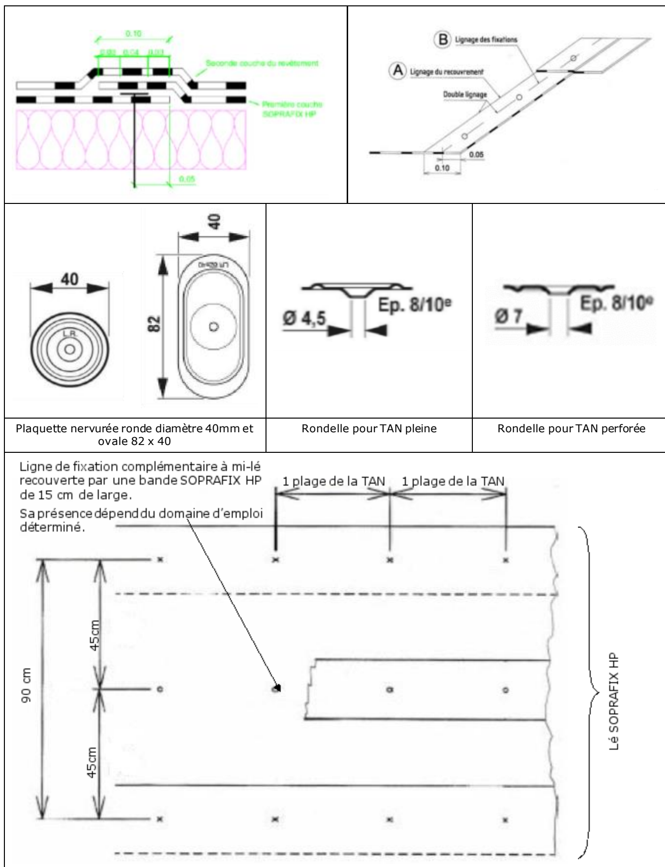
Figure 28 : Mise en œuvre du revêtement d'étanchéité avec première couche SOPRAFIX HP et plaquette de répartition
