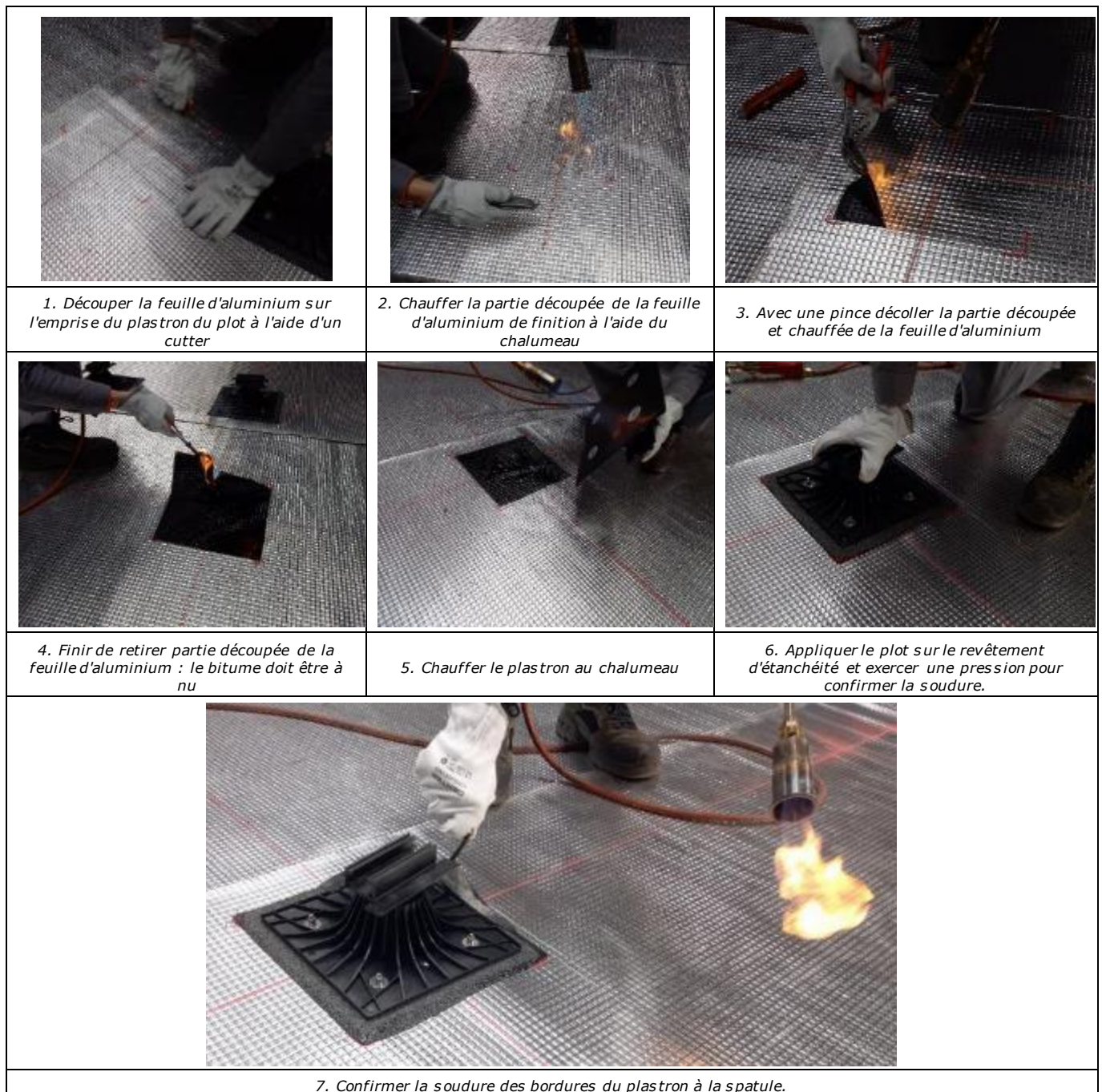
Figure 37 : Soudage des plots SOPRASOLAR FIX EVO sur membrane d'étanchéité avec finition aluminium SOPRALENE FLAM 180 ALU
