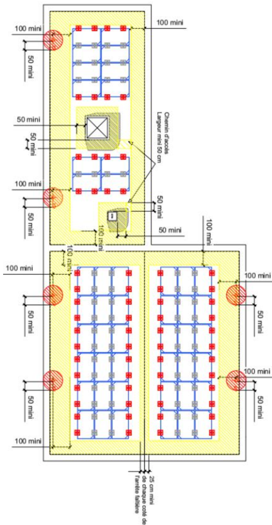
Figure 41 : Exemple calepinage standard (2 plots/grand côté du module) et préparation de la toiture en pose à plat
