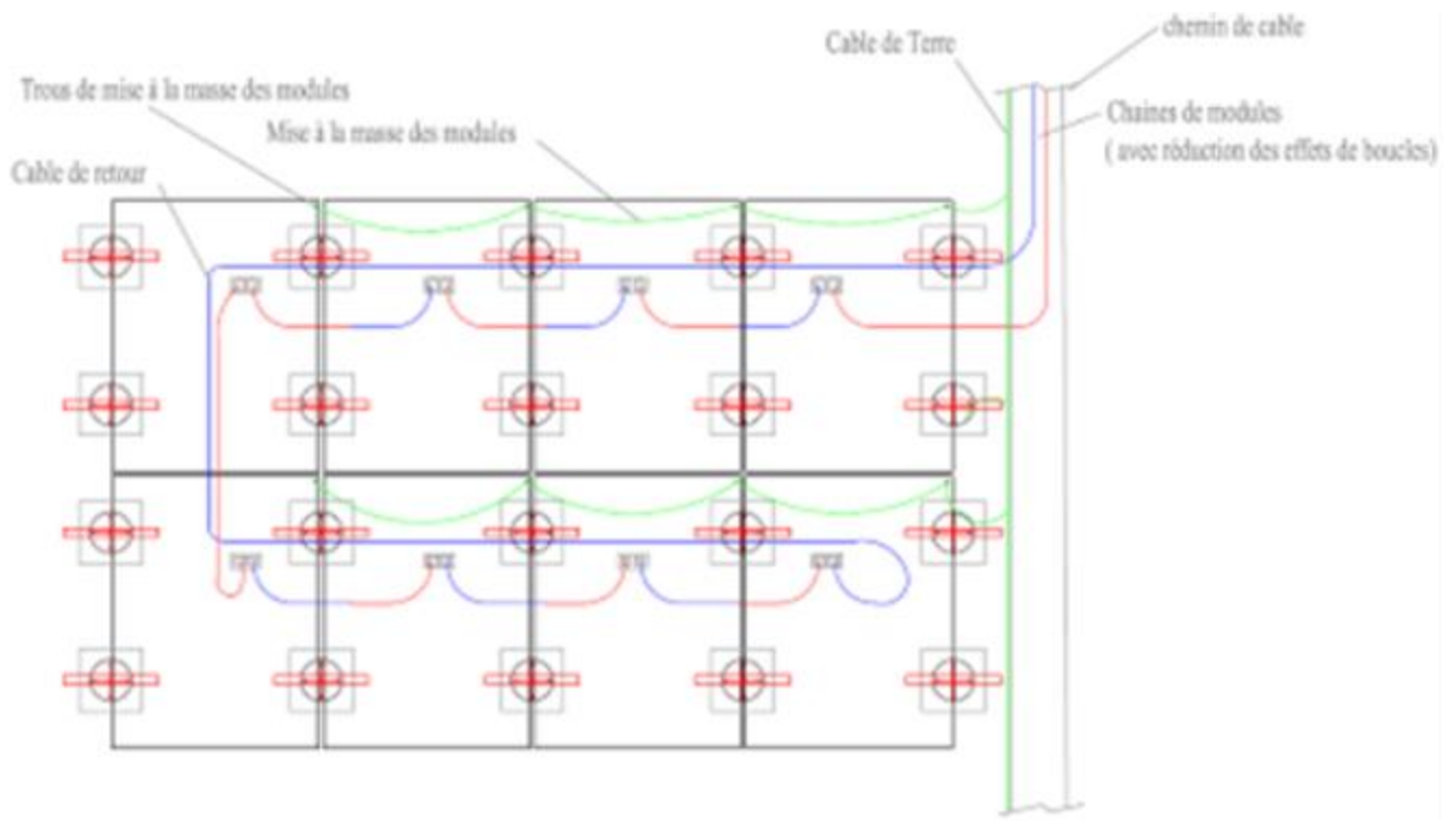
Figure 24 : Schéma de câblage et mise à la terre
