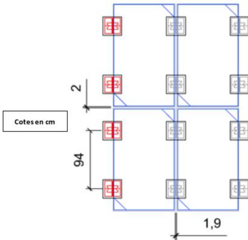
Figure 34 : Implantation des plots SOPRASOLAR FIX EVO en calepinage non densifié
