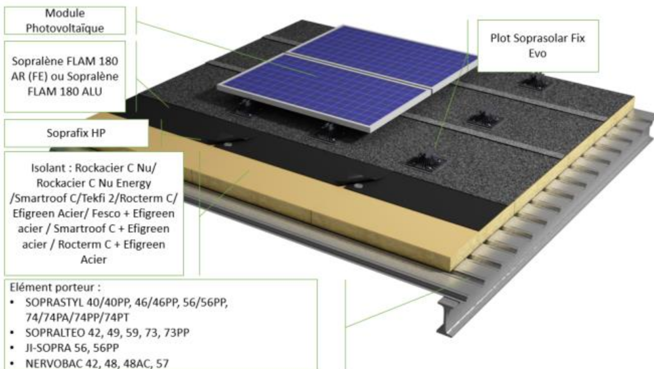
Figure 1 : Procédé en version SOPRASOLAR FIX EVO - TAN DTU sur élément porteur TAN avec revêtement d'étanchéité bicouche fixé mécaniquement et modules photovoltaïques
