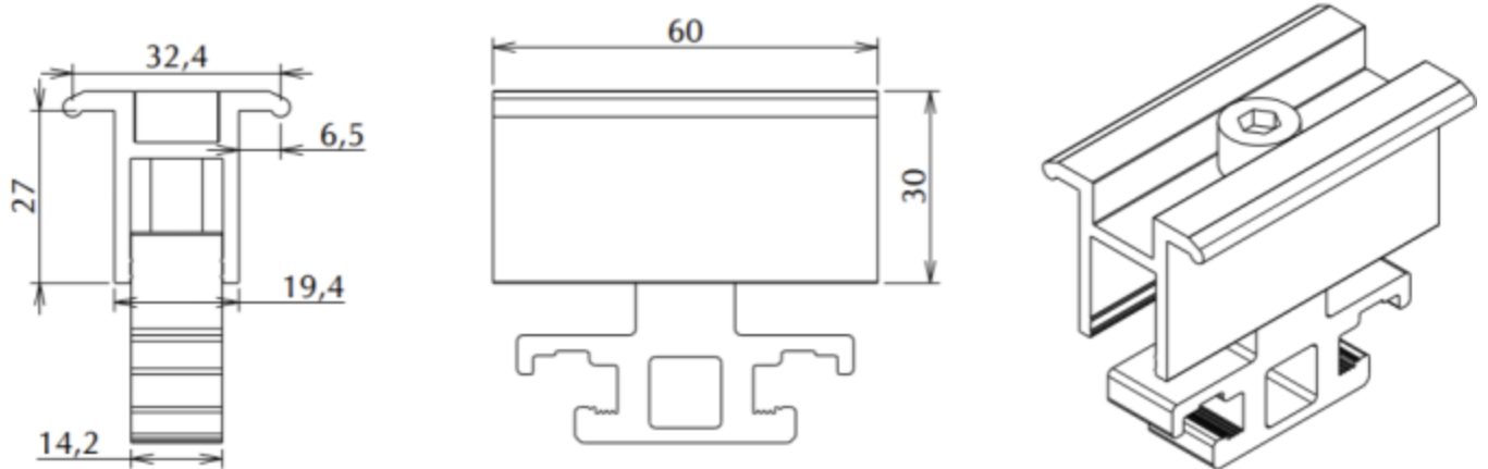
Figure 13 : Étrier universel STIB
