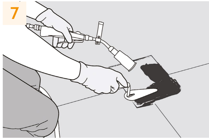
7 Noircir l'emplacement du plot à l'aide du chalumeau et d'une spatule.
