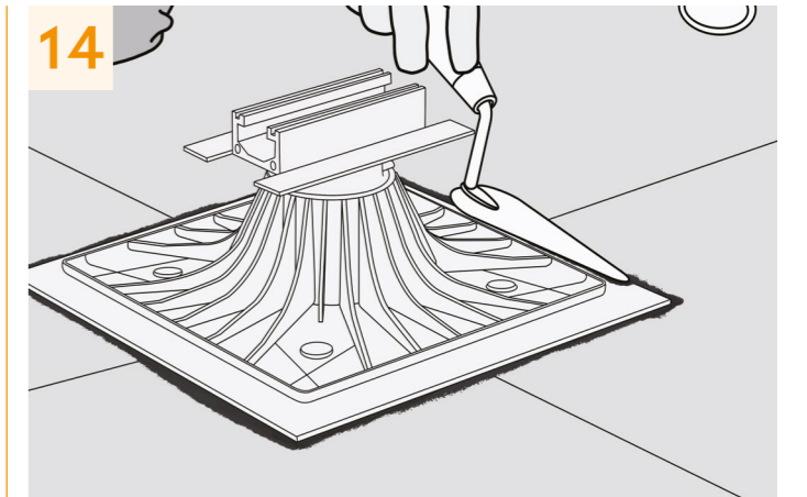
14 Confirmer la soudure des bordures du plastron à la spatule.
