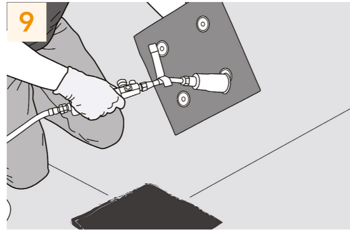
9 Brûler le film thermofusible à l'aide du chalumeau puis chauffer la face inférieure du plastron.
