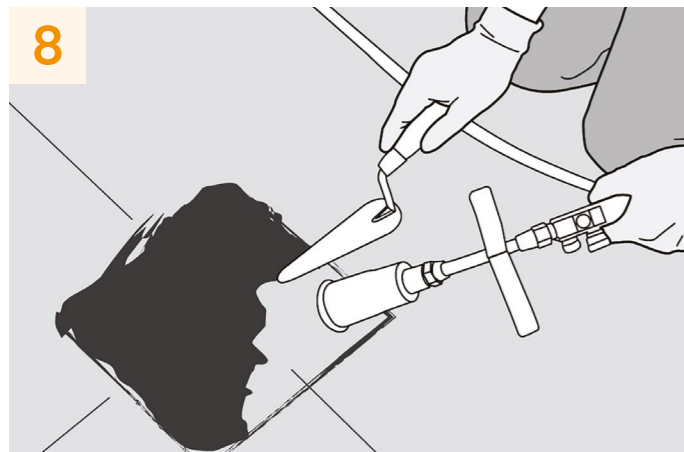
8 Dégréser les paillettes d'ardoises de la feuille d'étanchéité apparente.
