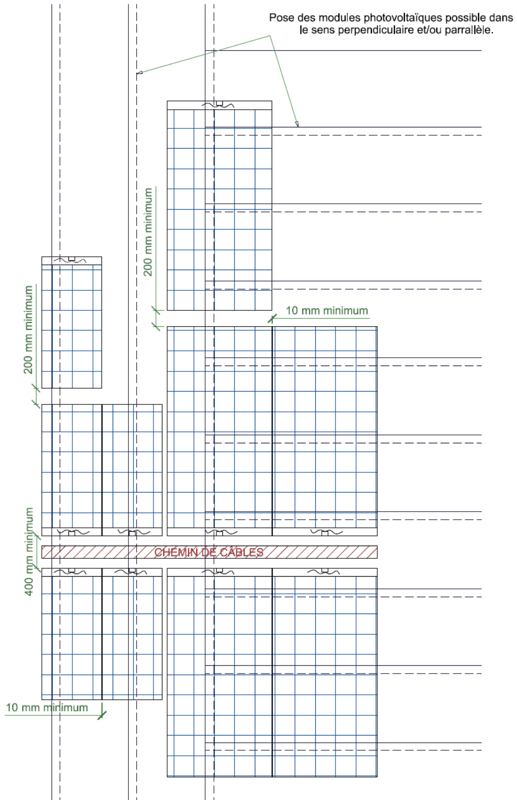
Figure 6 : Distances entre modules photovoltaïques pour le procédé SOPRASOLAR FLEX BITUME
