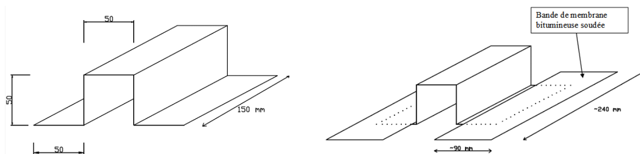
Figure 15 : Support de chemin de câble métallique
