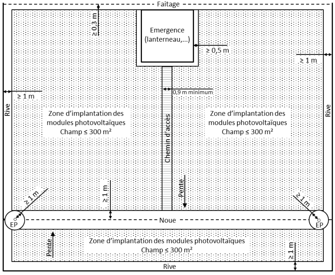
Figure 5 : Implantation des modules photovoltaïques
