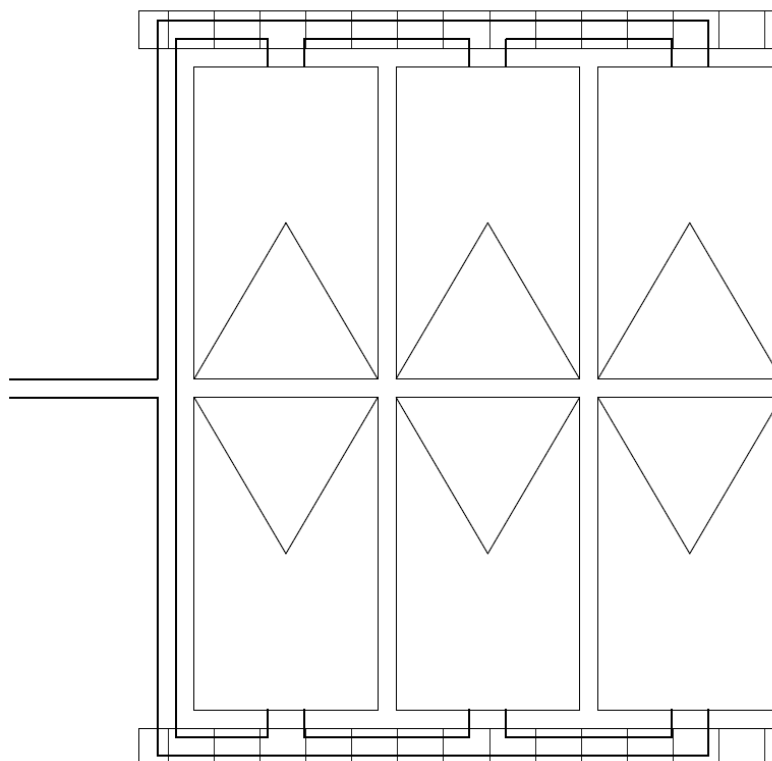
Figure 18 : Schéma de câblage des modules photovoltaïques
