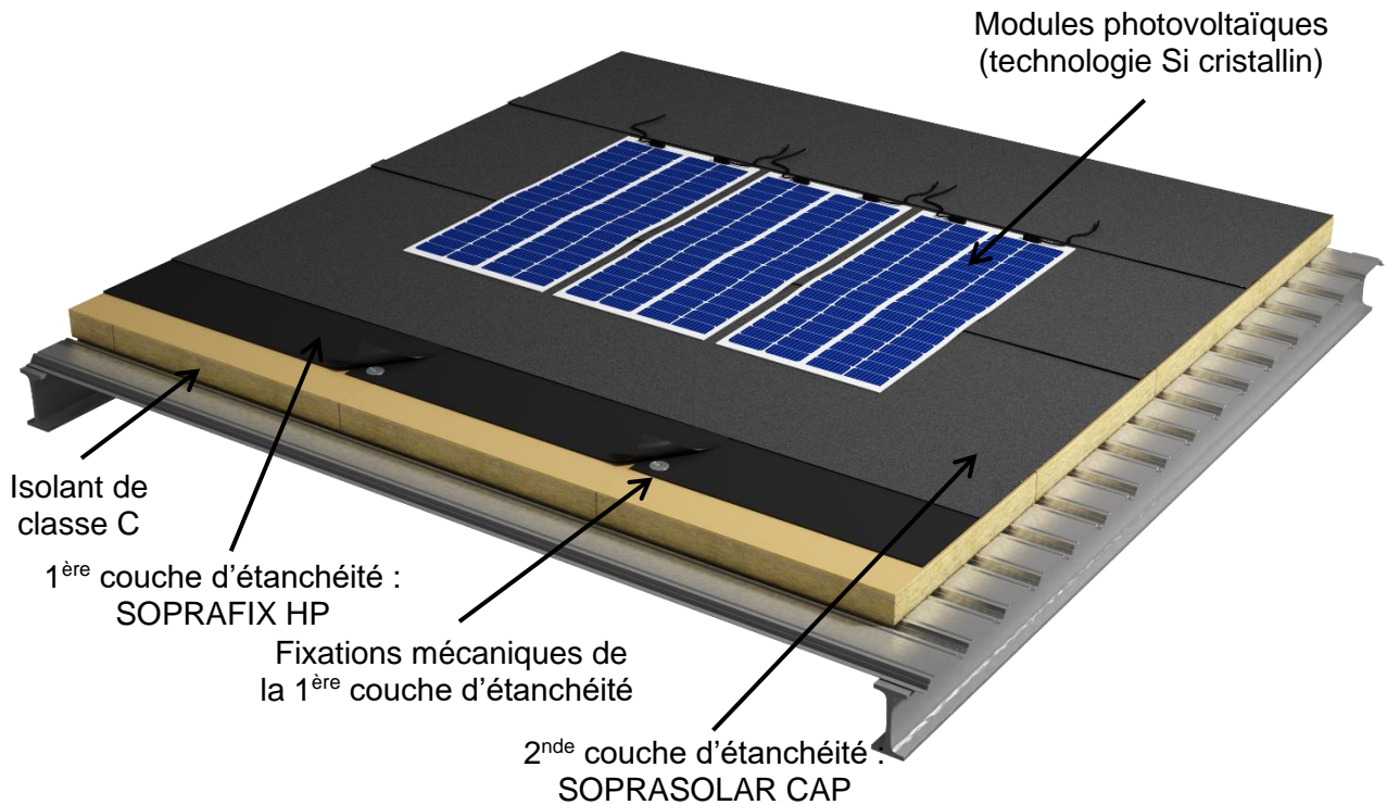
Figure 3 : Aperçus du procédé SOPRASOLAR FLEX BITUME sur revêtement d'étanchéité fixé mécaniquement (type F) – module PV parallèle aux rangées de fixations de l'étanchéité (SRA)
