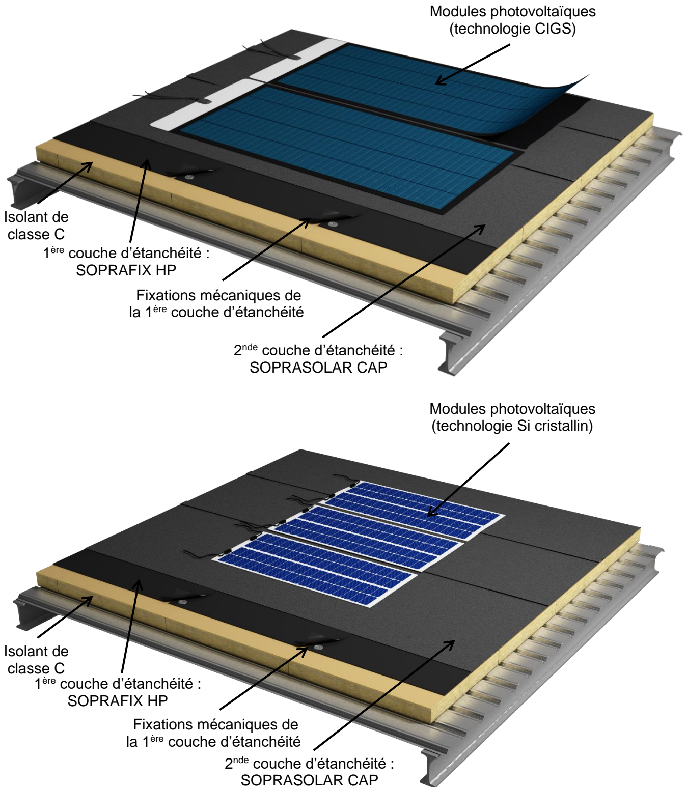
Figure 4 : Aperçus du procédé SOPRASOLAR FLEX BITUME sur revêtement d'étanchéité fixé mécaniquement (type F) – module PV perpendiculaire aux rangées de fixations de l'étanchéité (SRB)
