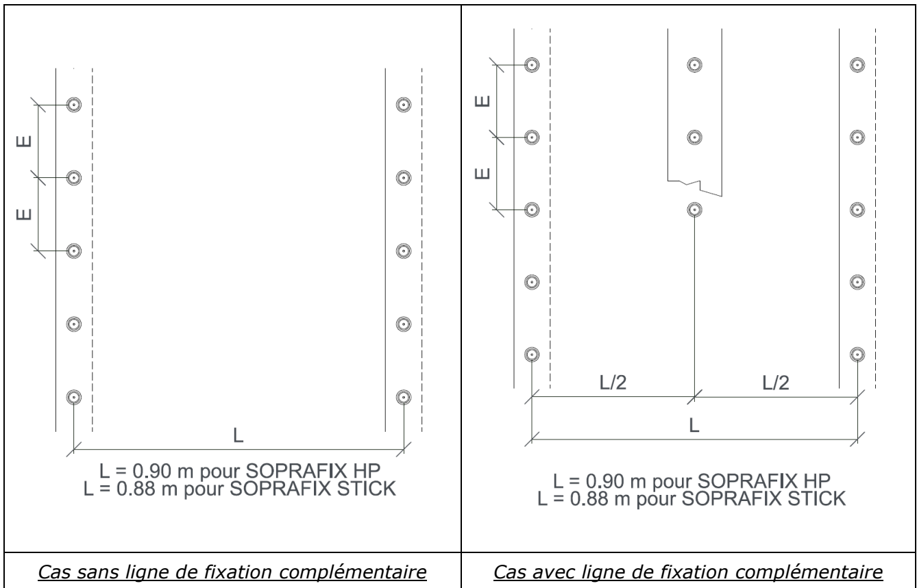
Figure 13 : Disposition des fixations de la première couche d'étanchéité
