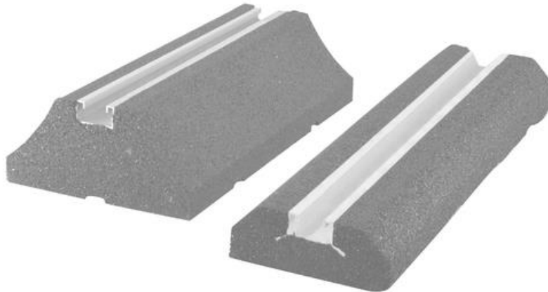
Figure 11 : Supports de chemin de câbles type "bigfoot"
